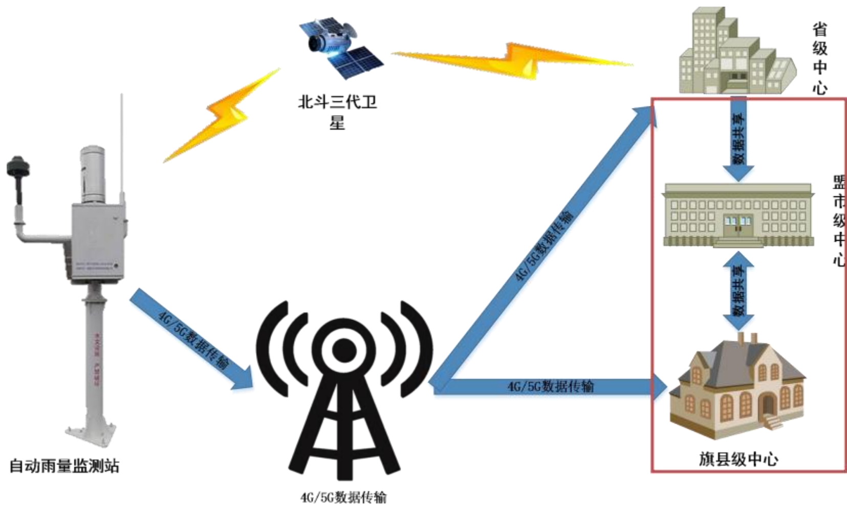
图 3-3-3 内蒙古自治区北斗终端通信管理架构框图
