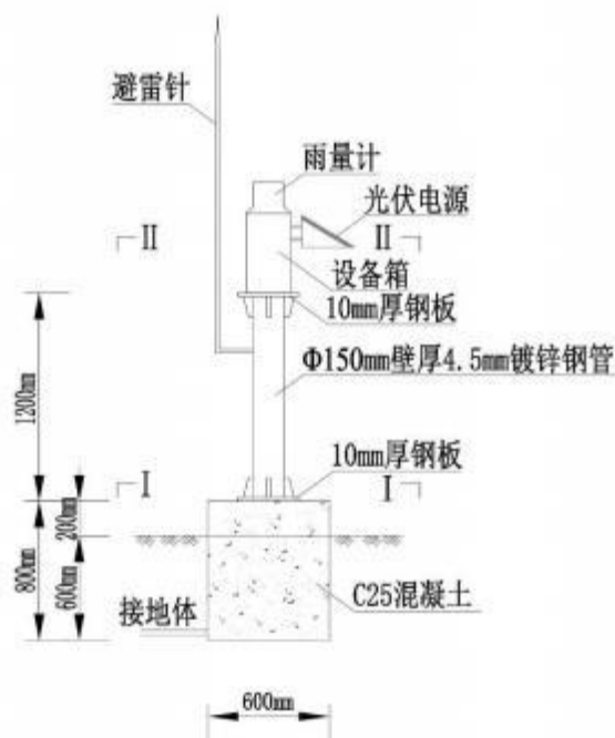
图 3-2-1 雨量站安装结构示意图
