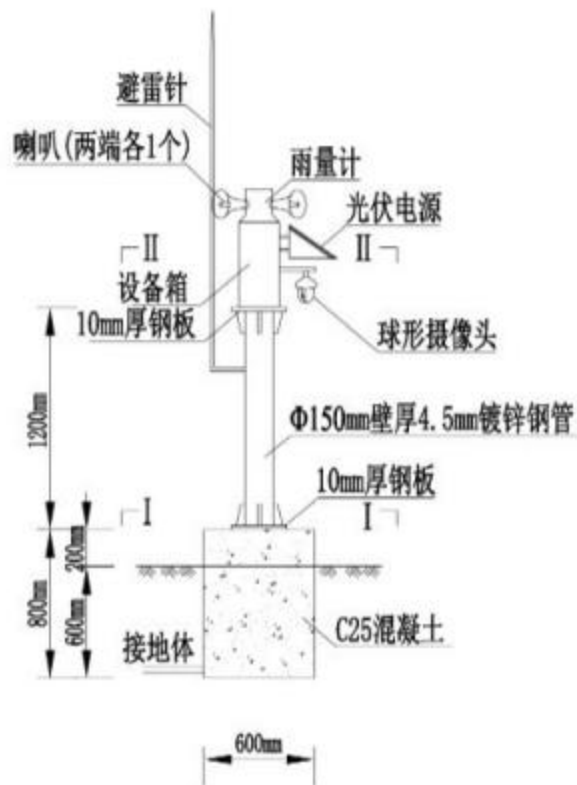
图 3-6-1 雨量站安装结构示意图
