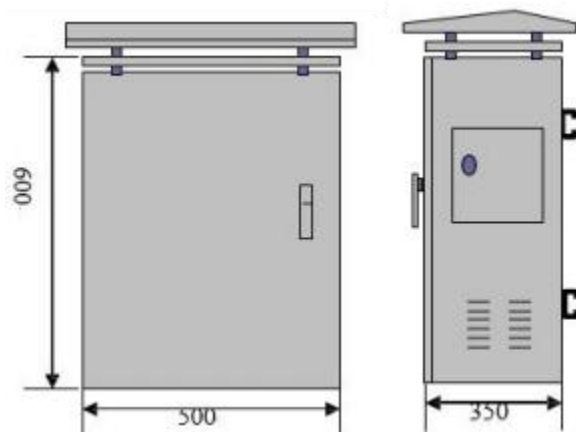
图 3-6-4 设备箱体
